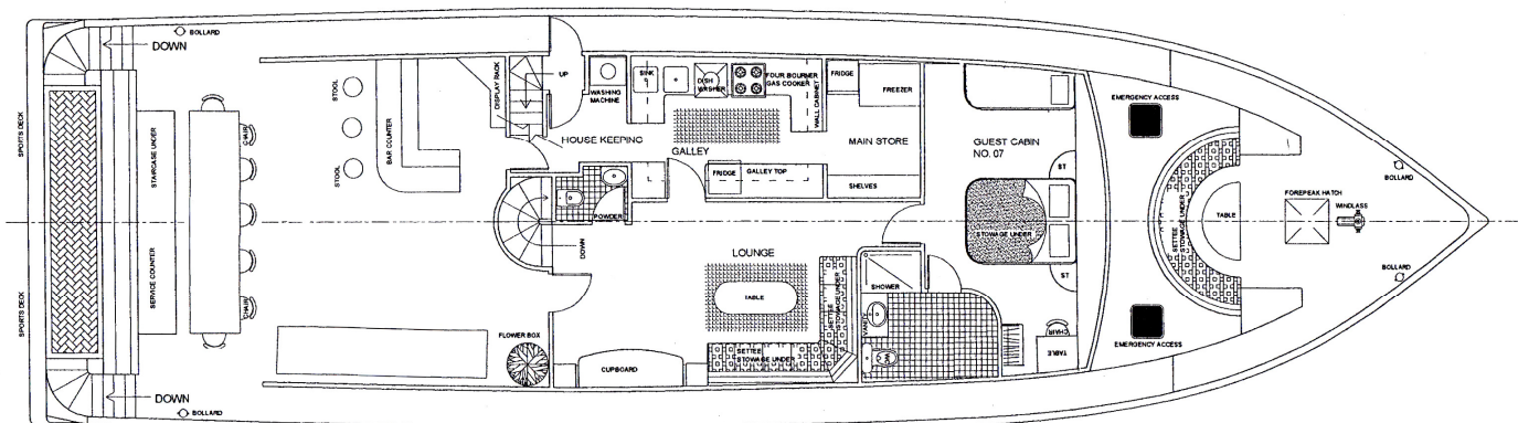
Piante del M/YACHT anastasia
